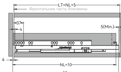
МОНТАЖ НАПРАВЛЯЮЩИХ С ВНУТРЕННИМ ФАСАДОМ
