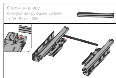
УСТАНОВКА СИНХРОНИЗИРУЮЩЕЙ ШТАНГИ
