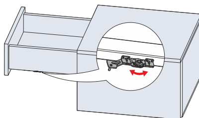
РЕГУЛИРОВКА ПО ГЛУБИНЕ
