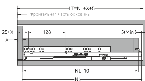
РЕГУЛИРОВКА ПО ГЛУБИНЕ
