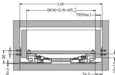
МОНТАЖ НАПРАВЛЯЮЩИХ С НАКЛАДНЫМ ФАСАДОМ
