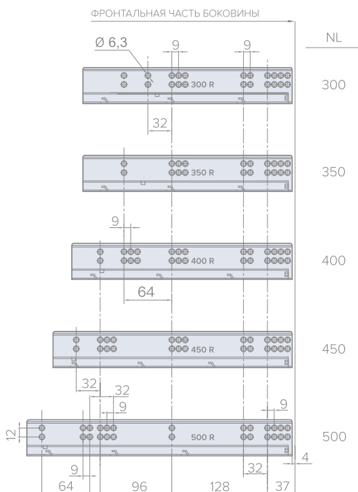
МОНТАЖ НАПРАВЛЯЮЩИХ
