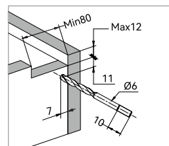
КРЕПЛЕНИЕ ЗАМКОВ И РЕГУЛИРОВКА ФАСАДА
